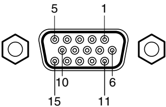
15-контактный разъем мини D-sub
