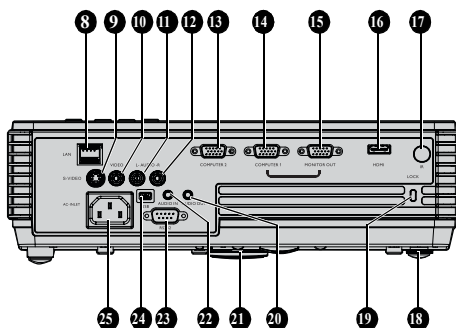
Вид снизу/сбоку
